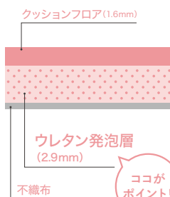
遮音フロア断面図
