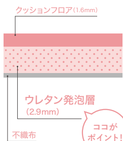
遮音フロア断面図
