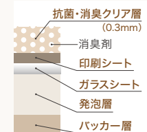
断面図 (3.0mm)
