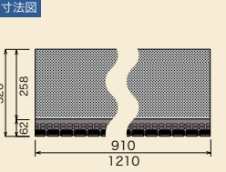
PX-5721 NEW (910mm 巾) PX-5722 NEW (1210mm 巾)
