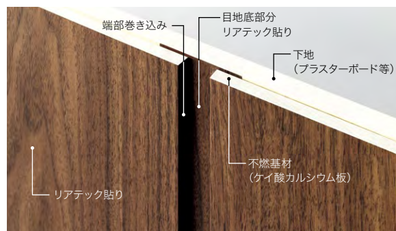
目透かし工法の断面図
