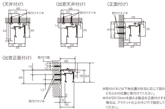
取付け寸法図(mm)
