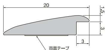
断面図 (単位:mm)
