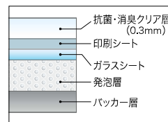
断面図(3.0mm)
