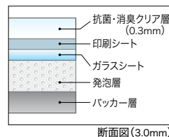
断面図(3.0mm)
