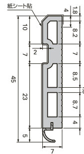
断面図 (単位:mm)
