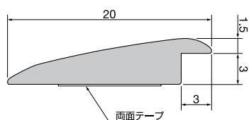
断面図 (単位:mm)
