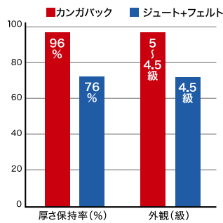
耐久性試験 (テトラポッドウォーキングテスト)
