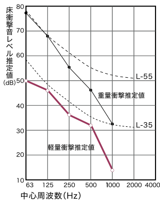
床衝撃音遮断性能試験
