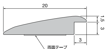
断面図 (単位:mm)
