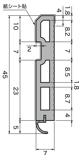
断面図 (単位:mm)
