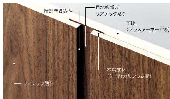
目透かし工法の断面図
