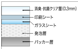
断面図 (3.0mm)
