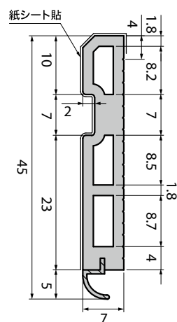
断面図 (単位: mm)
