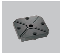
サポートパネル用 上部固定部材 83×83×H32mm GB-10313 ￥850/個 重量：約0.04kg
