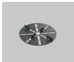
サポートパネル用 タイルフリースペース 167×167×H16mm GB-10315 ￥980/枚 重量：約0.07kg
