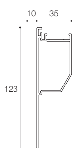
根太小口用幕板固定金具
