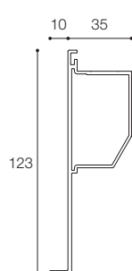
根太小口用幕板固定金具
