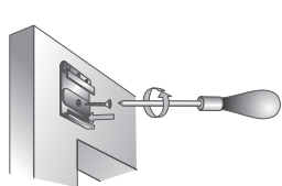
図1 正面付け
