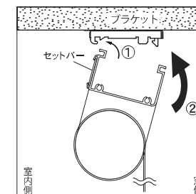
▲天井付け
