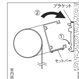
▲正面付け
