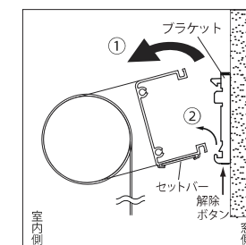
▲正面付け
