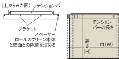
▲天井付け
