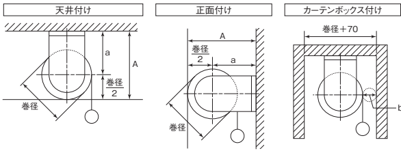
■標準T型・バス標準B型【製品巾 W2,000mm以下の場合】(単位：mm)
