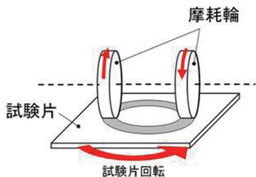
テーバー式磨耗試験機
