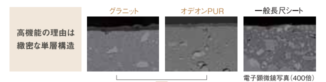
電子顕微鏡写真(400倍)
